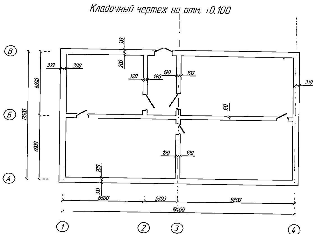
Рисунок 1. Кладочный чертеж
